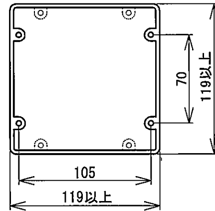
センサー取付用埋込BOX (別途)
