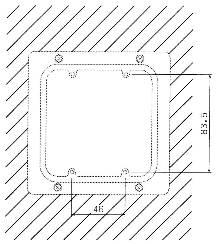
センサー金具取付寸法
