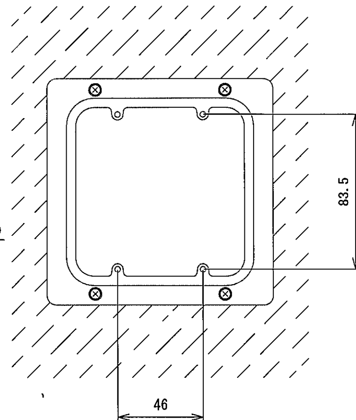
センサー金具取付寸法
