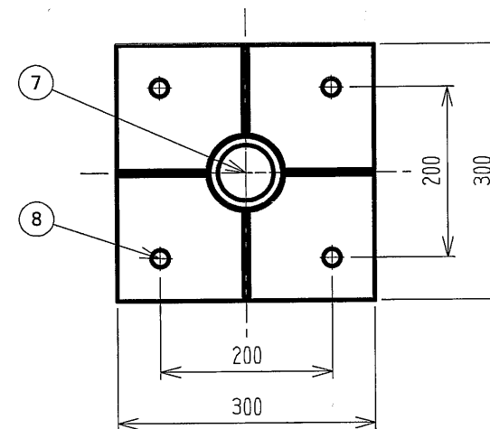
取付ベース詳細
