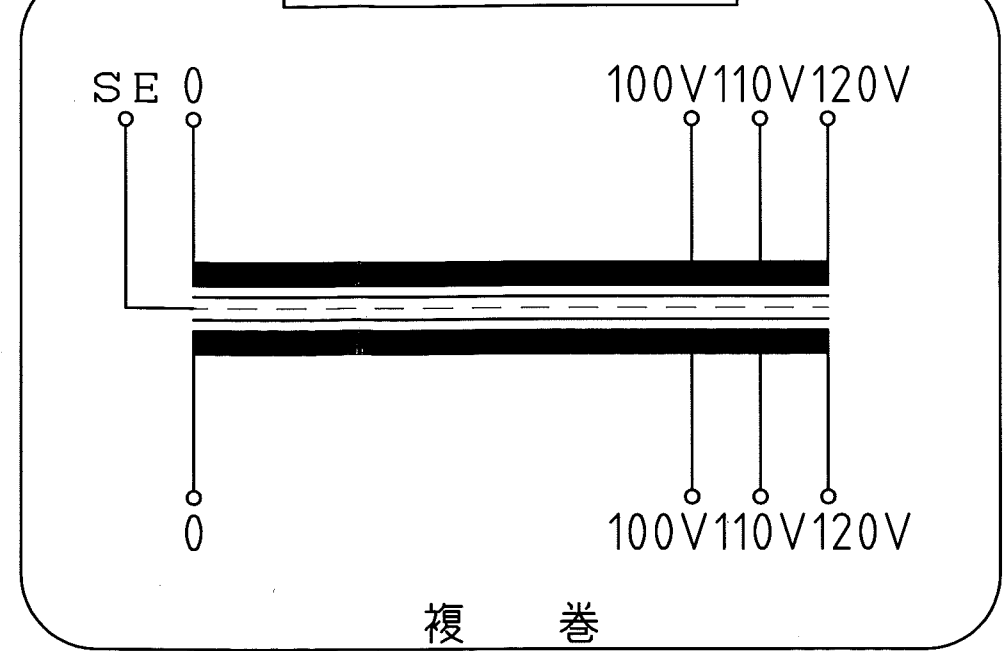
結線図
